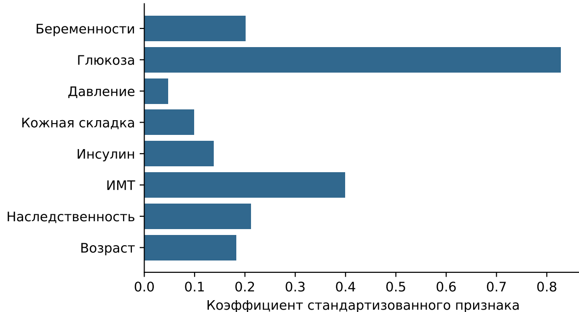
Выбранная модель
